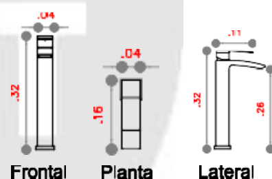
GRIFERIA LAVAMANOS ALTA KRIMML NEGRO 25479
